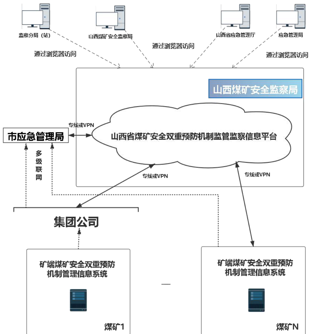
图 1 系统联网拓扑图
